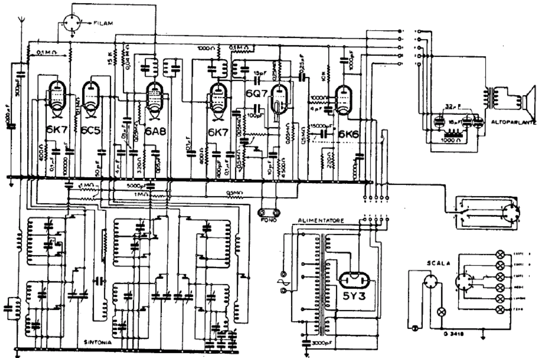
RADIO SUPERLA . MOD. « 751 »
